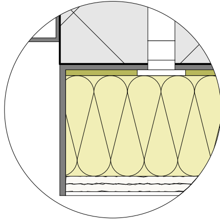
Aluminiumabschlusswinkel 2 mm
