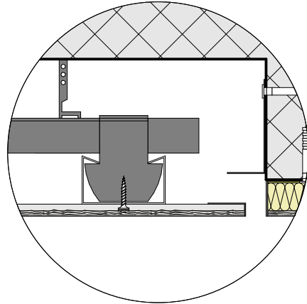
Systemaufbau
