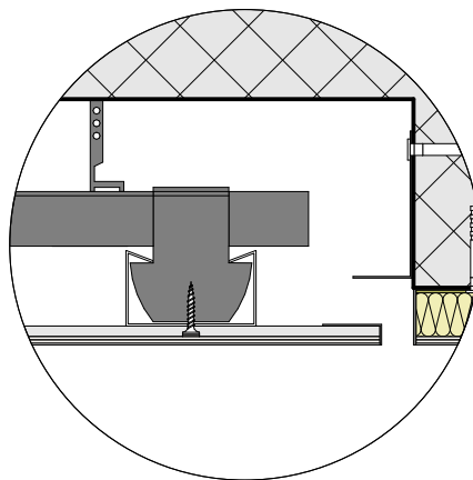
Systemaufbau
