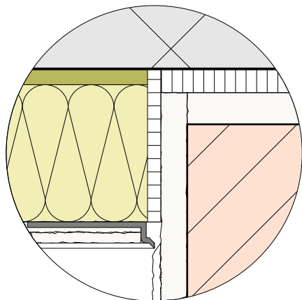
Acoustic Abschlussprofil
