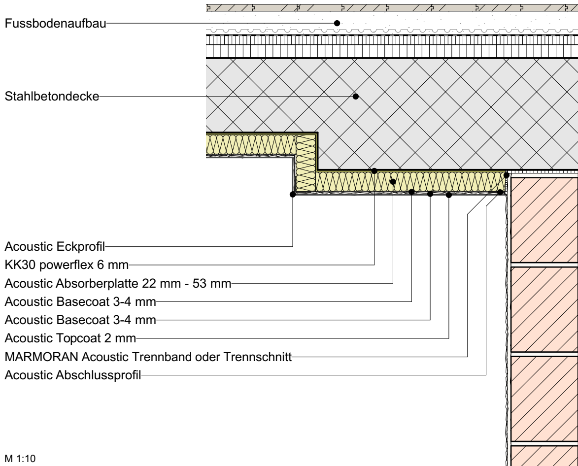
Acoustic Eckprofil
