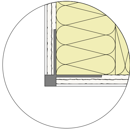
Acoustic Eckprofil
