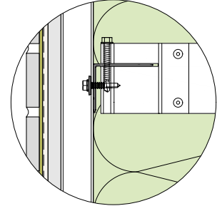
Systemschnitt Wand M 1:5
