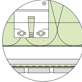
Systemschnitt Untersicht M 1:5
