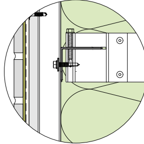
Systemschnitt M 1:5
