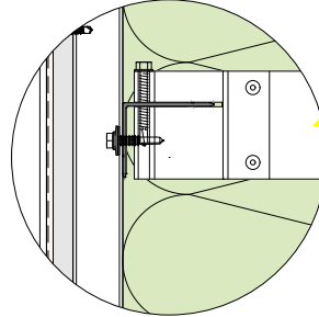
Systemschnitt M 1:5
