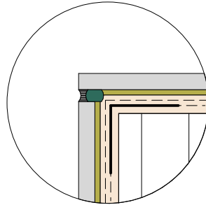
Gebäudeecke mit Fugenmörtel
