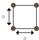
Dübelraster/Tabelle (Ceramo EPS/PIR/MW)
