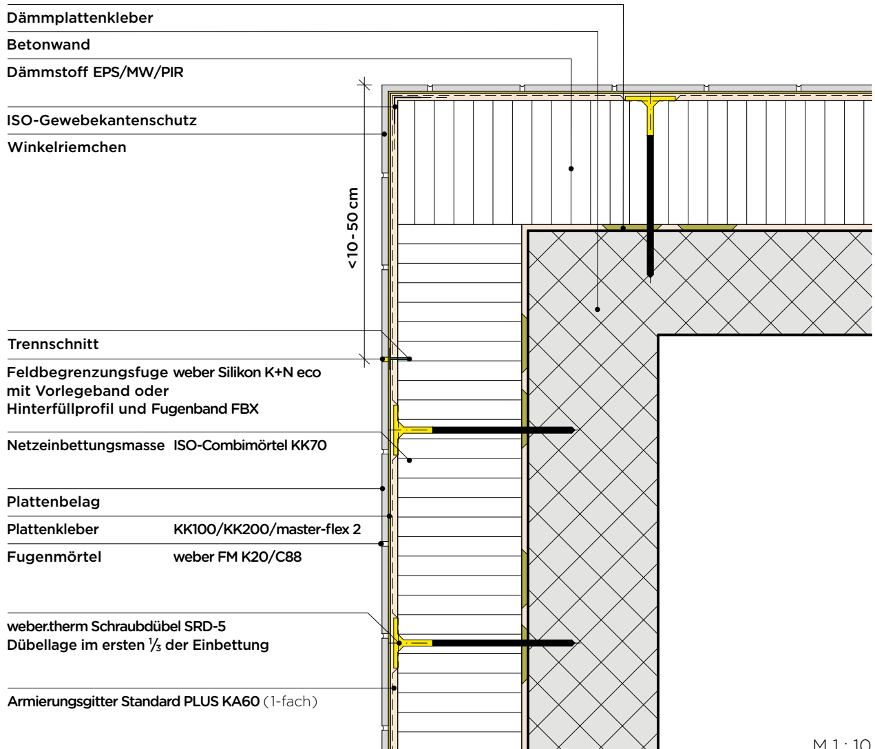
Variante werkseitig verklebt
